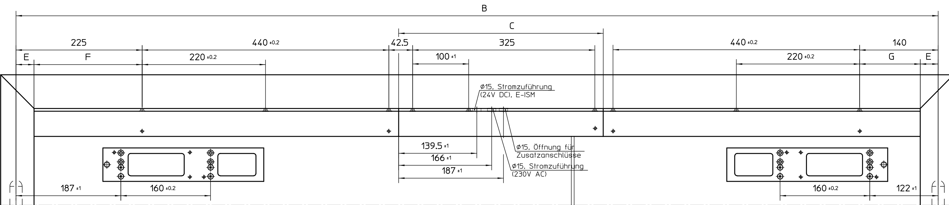
Anschlagmaß DIN rechts (Gangflügel)
