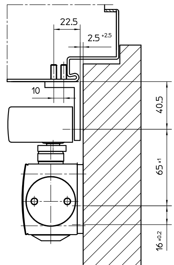
Anschlagmaß DIN rechts (Gangflügel)
