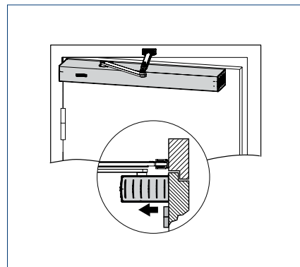
Türblattmontage mit Gestänge ECturn | Powerturn
