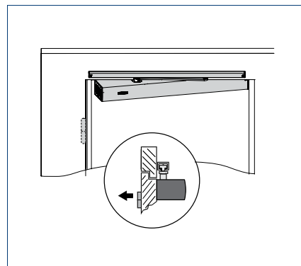
Türblattmontage mit Gleitschiene / Rollenschiene ECturn | Powerturn
