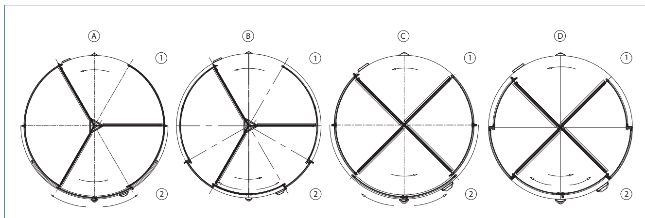
A = Dreiflügelig mit außenlaufendem Nachtverschluss | B = Dreiflügelig mit innenlaufendem Nachtverschluss | C = Vierflügelig mit außenlaufendem Nachtverschluss | D = Vierflügelig mit innenlaufendem Nachtverschluss | 1 = Innen | 2 = Außen
